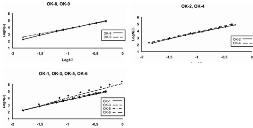
Şekil 3. Farklı bozunma derecelerine sahip 8 küçük örneğin fraktal boyutları.
