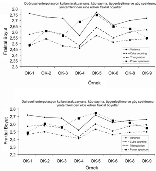
Şekil 5. Varyans, küp sayma, üçgenleştirme ve güç spektrumu yöntemlerinden elde edilen fraktal boyutların karşılaştırması
