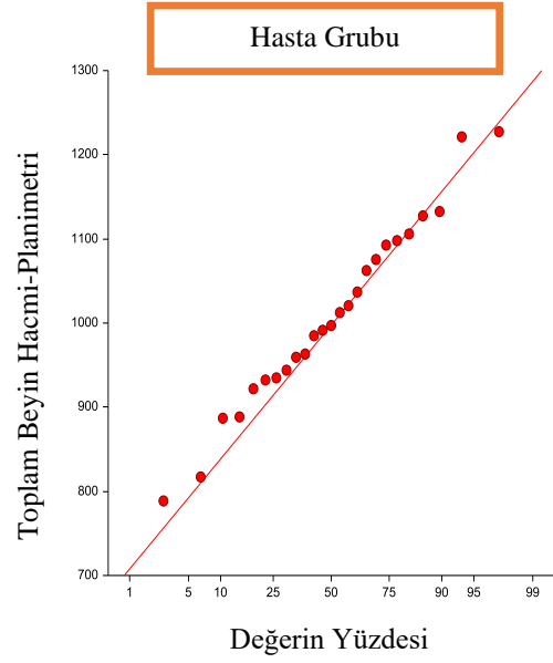
Şekil 4.37. Hasta grubunda Planimetri yöntemi ile ölçülen toplam beyin hacminin yüzdelik dağılım grafiği.
