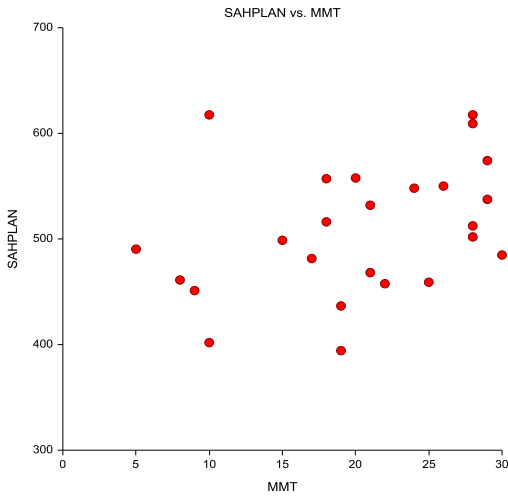
Şekil 4.7. Planimetri yöntemi ile ölçülen sağ beyin hemisfer hacminin MMT ile korelasyon grafiği.
