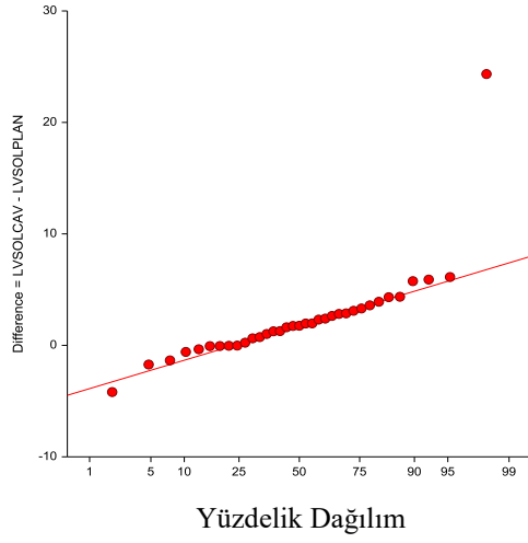
Şekil 4.127. İki yöntem arasındaki hacim farkı ortalamasının yüzdelik dağılım grafiği.
