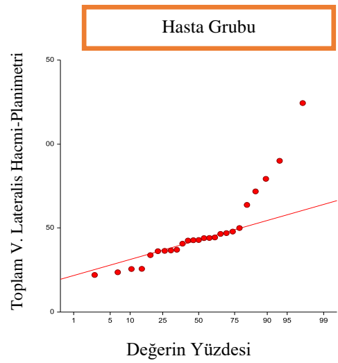
Şekil 4.52. Hasta grubunda Cavalieri yöntemi ile ölçülen toplam ventriculus lateralis hacminin yüzdelik dağılım grafiği.
