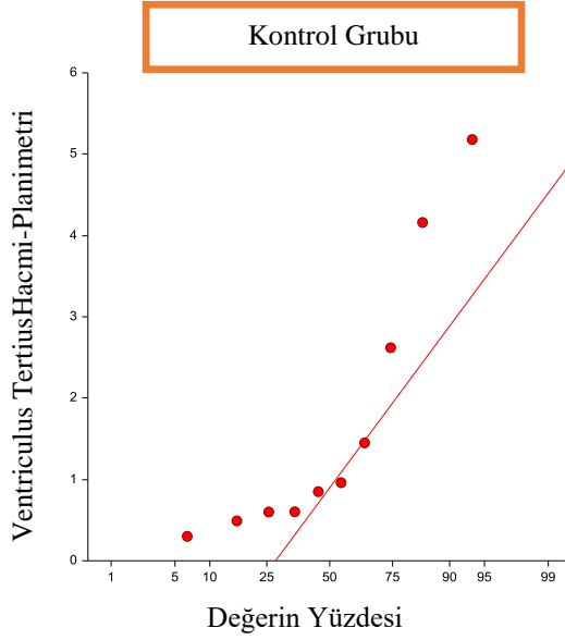
Şekil 4.72. Kontrol grubunda Planimetri yöntemi ile ölçülen ventriculus tertius hacminin yüzdelik dağılım grafiği.
