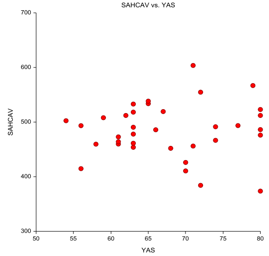
Şekil 4.6. Cavalieri yöntemi ile ölçülen sağ beyin hemisfer hacminin yaş ile korelasyon grafiği.
