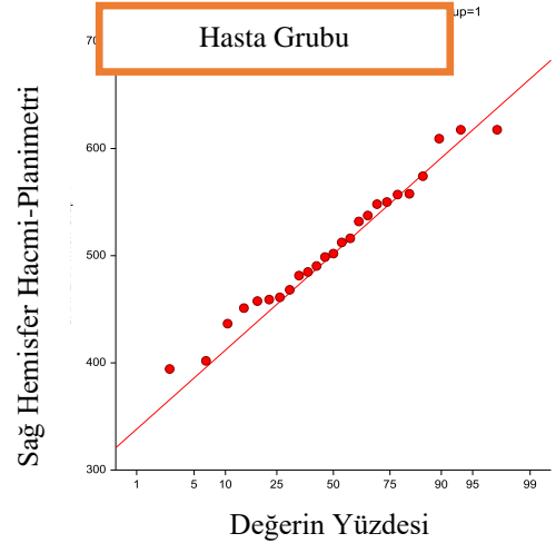
Şekil 4.43. Hasta grubunda Planimetri yöntemi ile ölçülen sağ beyin hemisfer hacminin yüzdelerik dağılım grafiđi.
