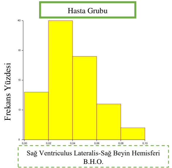
Şekil 4.85. Planimetri yöntemine göre hasta grubunda sağ ventriculus lateralis bileşen hacim oranları frekans yüzdesi. B.H.O. Bileşen Hacim Oranı
