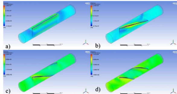
Fig. 6. Pressure vs roughness of 0.066 (a=0°, b=90°, c=180°, d=270°)
