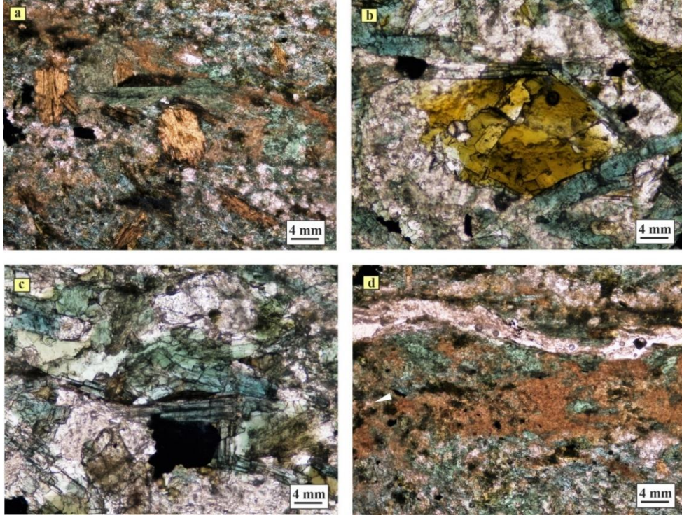
Şekil 4.12: (a) klorit-biyotit birlikteliği, (b) hornblend fenokristalini sarmalayan kloritlerin görünümü, (c) prizmatik klorit mineralleri, (d) kayalardaki karbonatlaşmanın genel görünümü (4X; Ç.N.).
