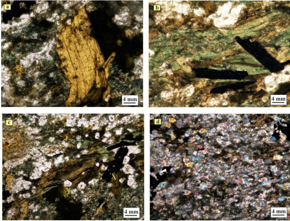
Şekil 4.13: (a) Metamorfizma etkisiyle kıvrımlanma gösteren biyotit (10X; Ç.N.), (b, c) sönme durumdaki biyotitler ve yeşil renkli kloritler, (d) yüksek girişim renkli özşekilsiz epidotlar (4X; Ç.N.).
