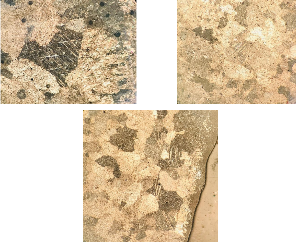
Şekil 4.2: Kalsit minerallerinin grift görünümleri ve tipik hasır ikizlenmeleri (10X; Ç.N.).
