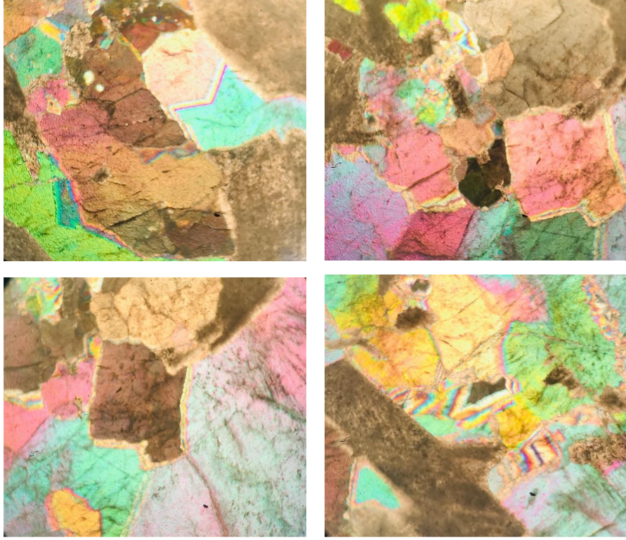
Şekil 4.4: Başalan mermerleri içerisindeki epidot minerallerinin çapraz nikol altındaki görünüşleri (4X).
