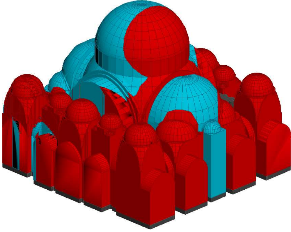
Şekil 5.35: 3d cisim kuzey yönünden perspektif
