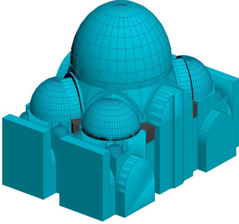
Şekil 5.83: 3d cisim kuzey yönünden perspektif
