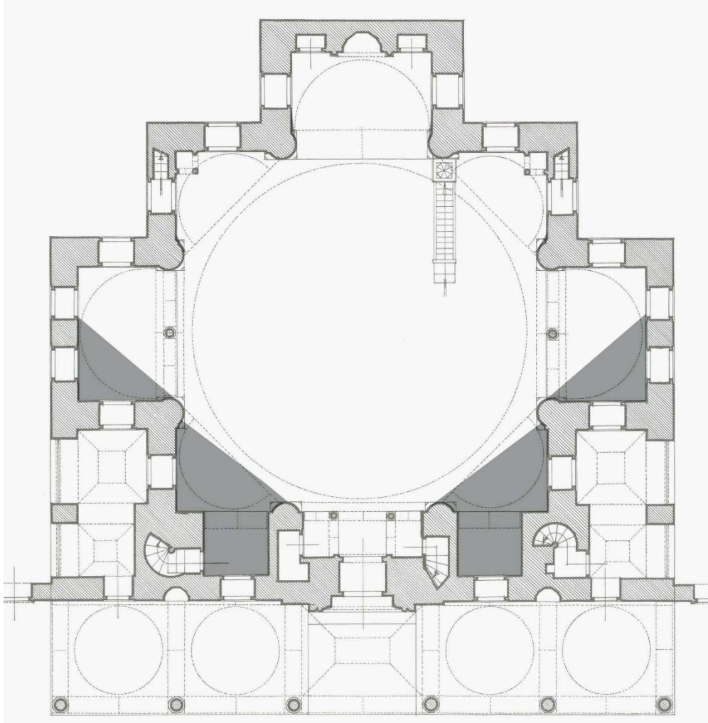
Şekil 5.102: Nişancı Mehmet Paşa Camii algılanabilir alanlar (Plan Ali Saim Ülgen'den alınmıştır)
