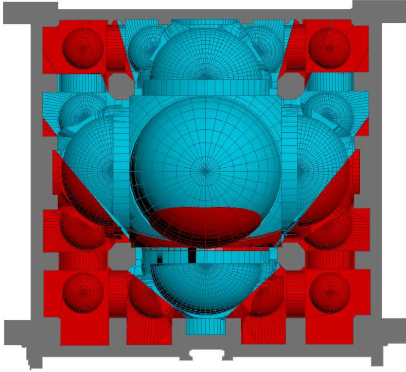
Şekil 5.19: 3d cisim üst görünüş
