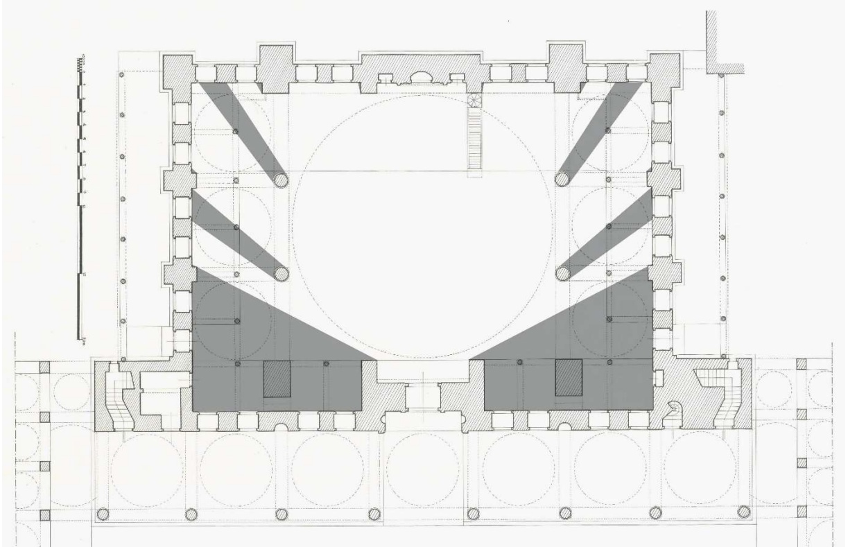
Şekil 5.66: Mihrimah Sultan Camii algılanabilir alanlar (Plan Ali Saim Ülgen’den alınmıştır)
