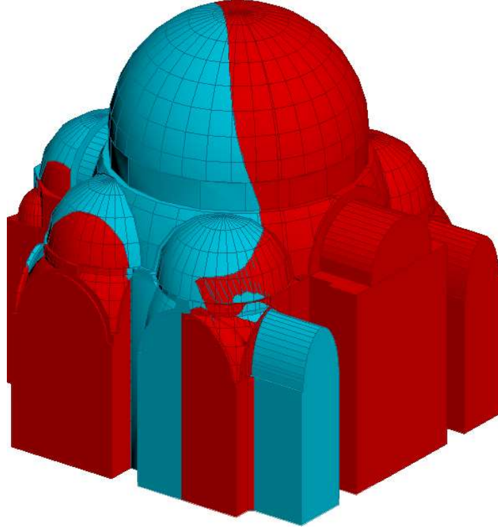
Şekil 5.125: 3d cisim kuzey yönünden perspektif
