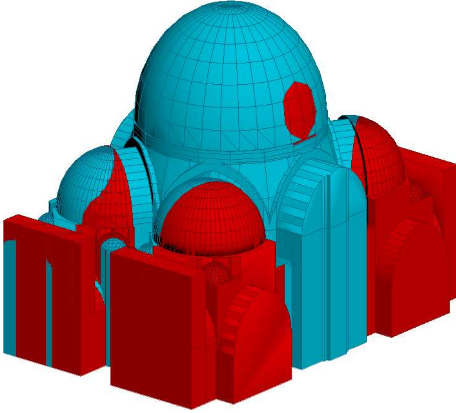
Şekil 5.89: 3d cisim kuzey yönünden perspektif
