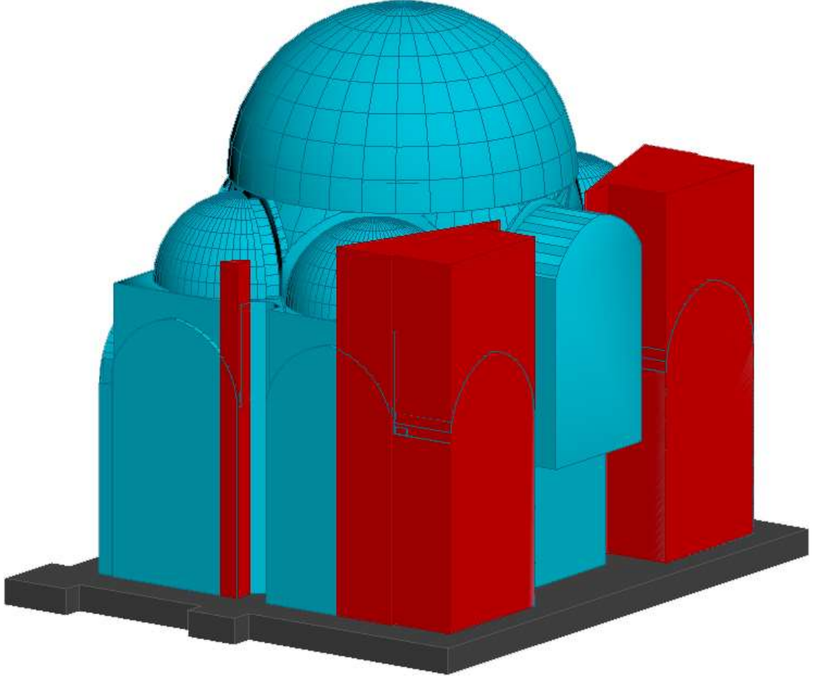
Şekil 5.97: 3d cisim kuzey yönünden perspektif
