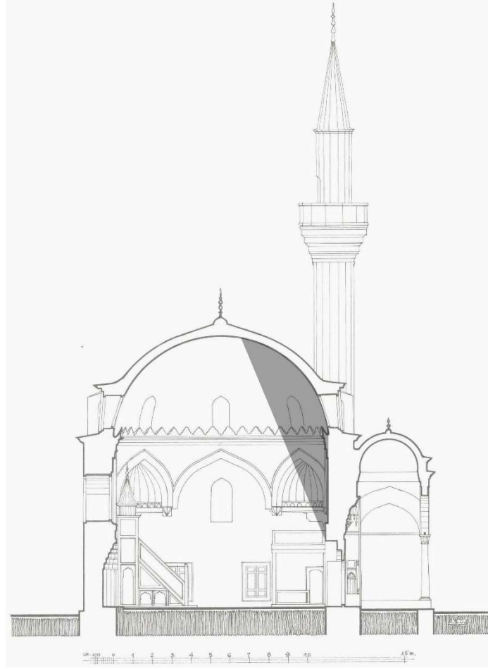
Şekil 5.2: Haseki Camii algılanabilir alanlar (Kesit Ali Saim Ülgen'den alınmıştır).
