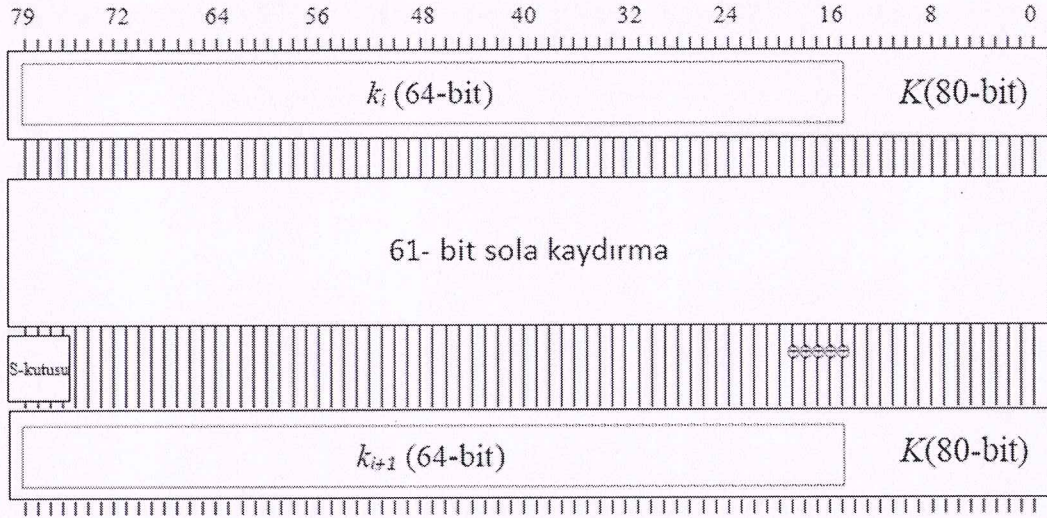
Şekil 2.2: Anahtar üretme algoritması.
