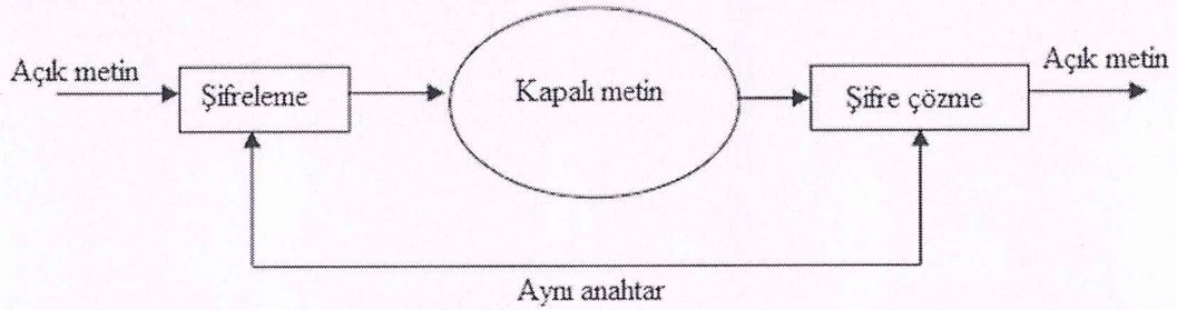
Şekil 1.1: Simetrik şifreleme.
