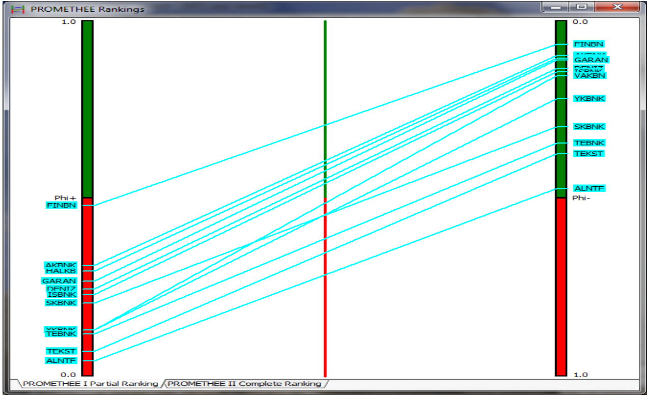
Şekil 2. 2011 Yılı İçin PROMETHEE I Sıralama Sonuçları
