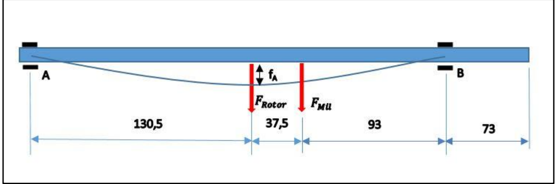
Şekil 2.17: Alternatör mili rotor orta noktasındaki sehimini.
