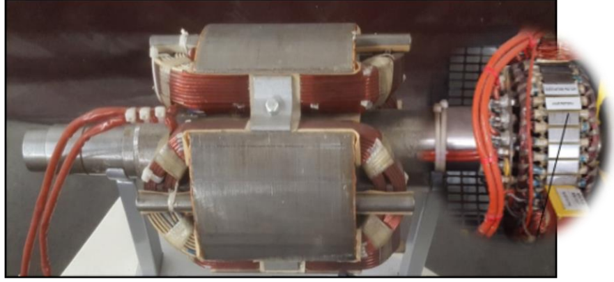
Şekil 1.4 : Alternatörün rotoru ve döner diyot.
