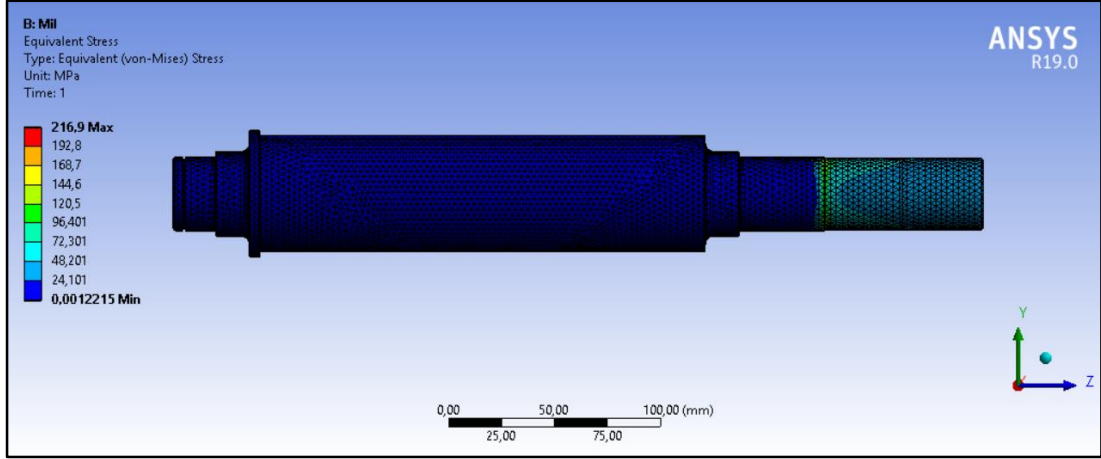
Şekil 2.24: Von-Misses gerilme.
