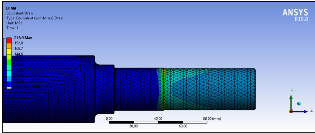
Şekil 2.25: Von-Misses gerilme bölgesi.
