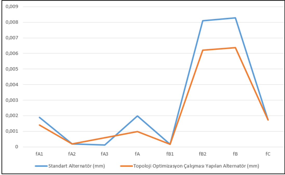
Şekil 4.2 Optimizasyon sonrası mil sehim farkları.
