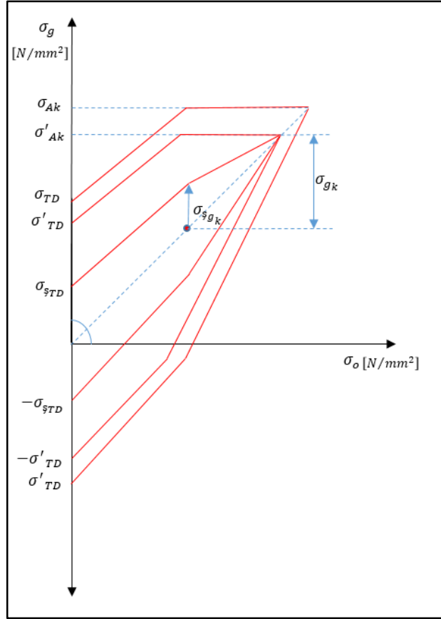
Şekil 2.10: Sürekli Mukavemet Diyagramı gösterimi [38].
