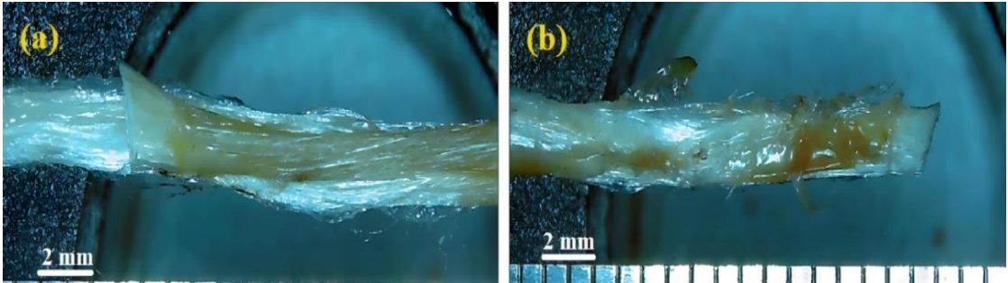
Şekil 6.53: CE600/TPU ipin (a) kaynak ve (b) sıyrılma/kopma bölgesi
