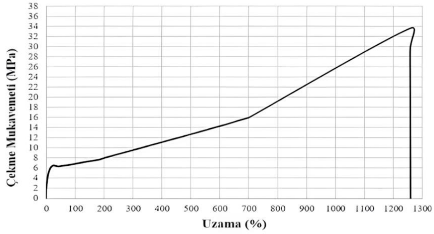
Şekil 6.8: TPU filamentin çekme mukavemeti – uzama (%) eğrisi
