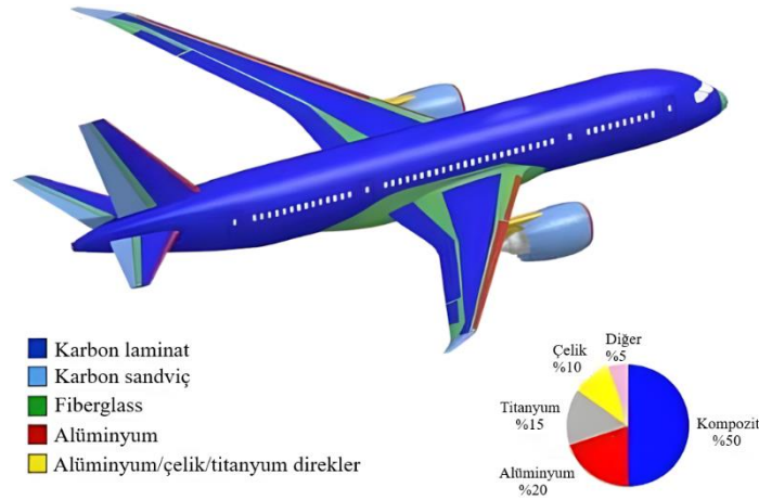
Şekil 2.3: Yolcu uçaklarında kullanılan malzemeler (Zhang Hongyu., 2019)
